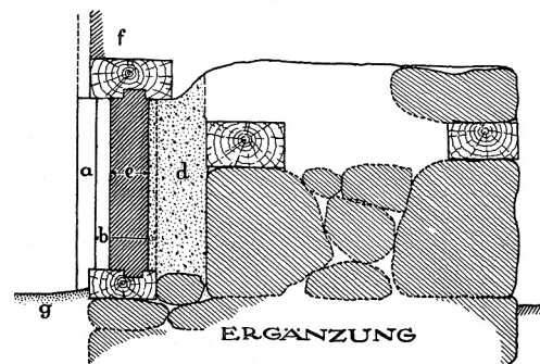
α -PARASTAS, b -ALABASTER-TRIGLYPH, c -GEBRANNTER ERDMÖRTEL, d -ERDMÖRTEL, e -METOPE, f -WAND, g -STUCK.
